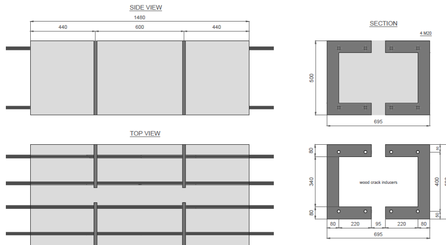
Figura 2 – Geometria provini tipo Y2, Y4
