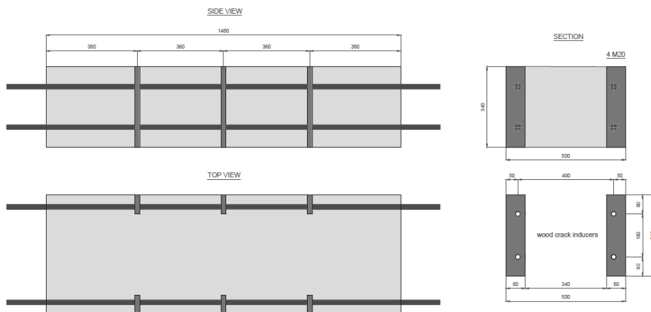
Figura 1 – Geometria provini tipo Y1a, Y1b
