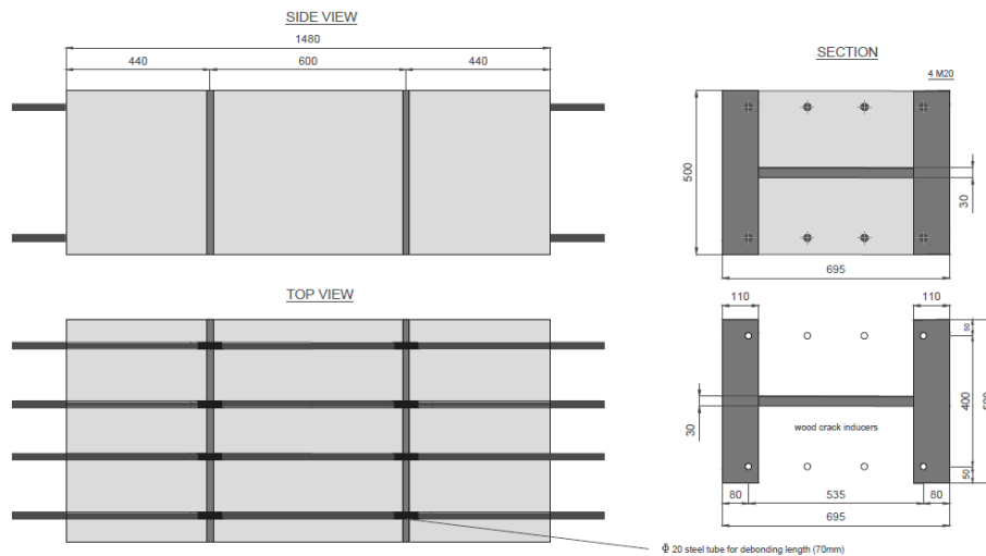
Figura 2 – Geometria provini tipo Y2, Y4
