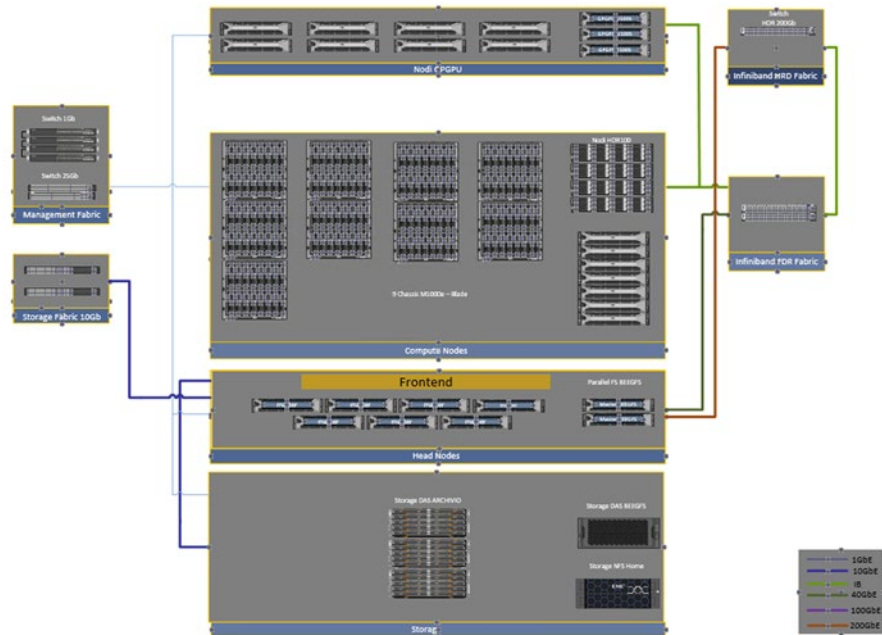
Figura 1 - Schema situazione attuale
