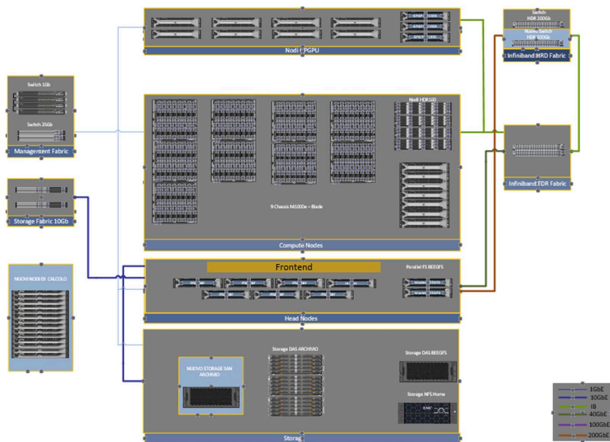
Figura 2 - Schema soluzione prevista
