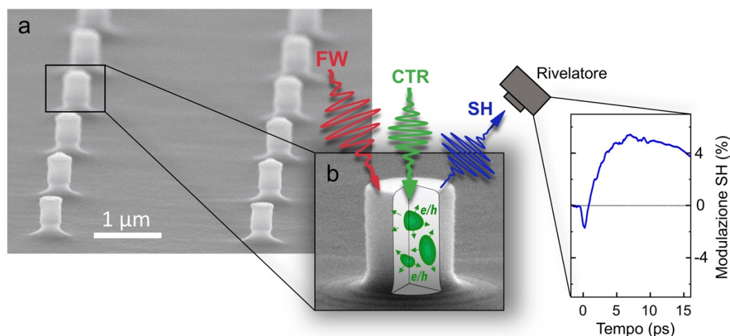
Figura 1. (a) Immagine al microscopio elettronico di nanoantenne ottiche nonlineari di arseniuro di gallio e alluminio. (b) Esperimento di riconfigurazione tutta-ottica di una nanoantenna nonlineare: un impulso di luce infrarosso (FW) genera luce visibile (SH), che viene riemessa dall’antenna modulata nel tempo grazie all’eccitazione di elettroni e lacune (e/h) prodotte da un impulso laser di controllo (CTR).
